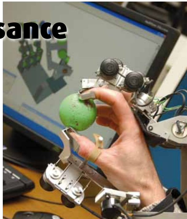
L'équipe RobiOSS travaille sur la préhension des machines : leur capacité à saisir et manipuler les objets.
